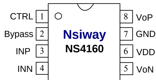
图2 eSOP8 装管脚分配图(top view)
