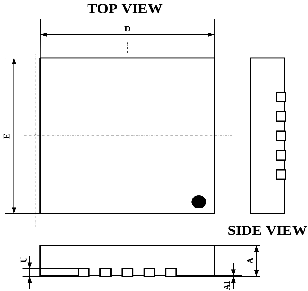
图 8-1 顶视图
