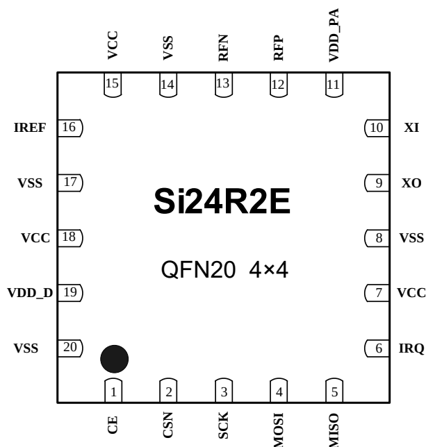
图 2-1 Si24R2E 引脚信息图（QFN20 4×4 封装）
