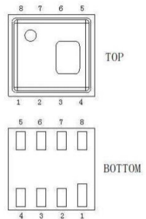
图 2：引脚图
