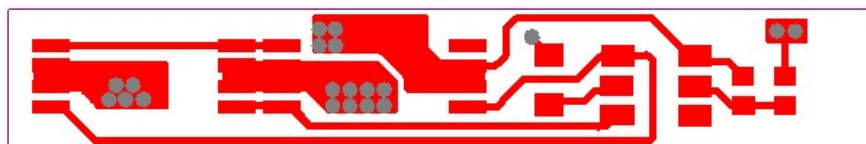
TOP SIDE
