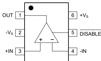
SOT-23-6
