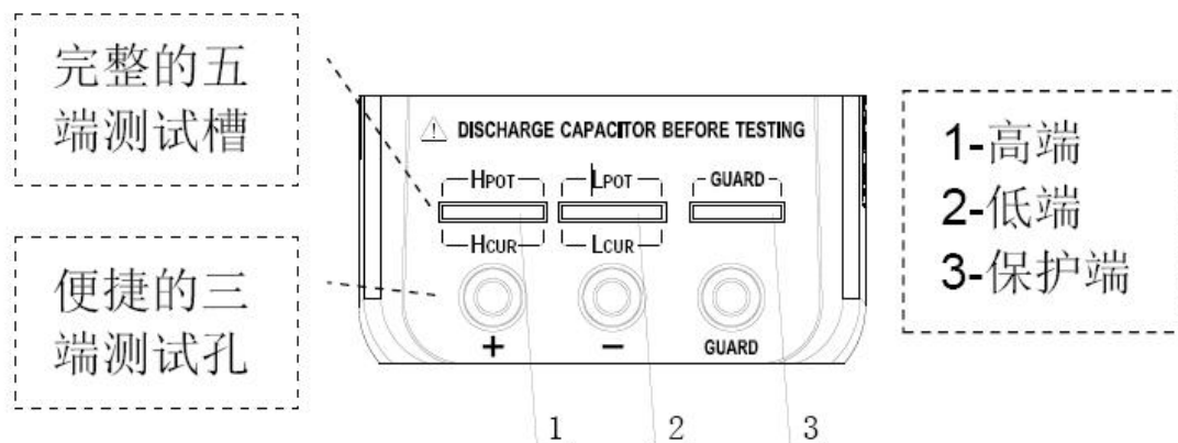
图 4 测试端口
