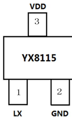
SOT-23-3
